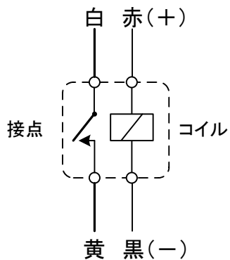
回路図
