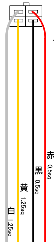
ソケット 下から見た図
